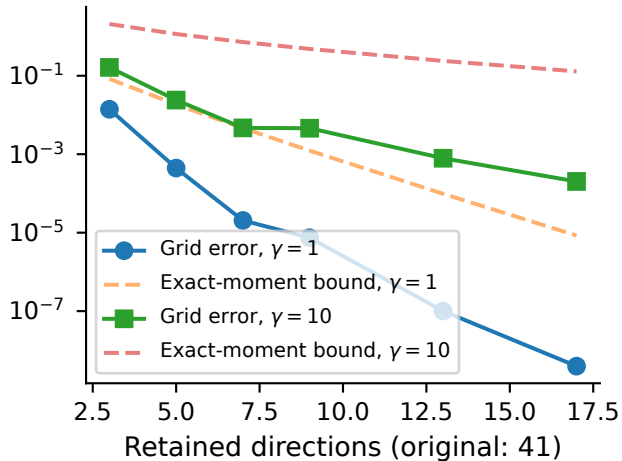
Information error (nats)
