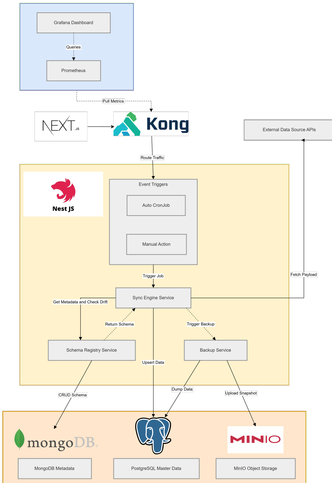
Hình 3.2: Tương tác giữa các module backend và với các thành phần bên ngoài
