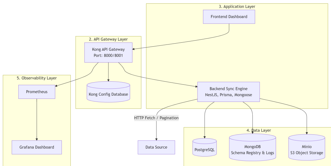
Hình 4.1: Sơ đồ kiến trúc tổng thể
