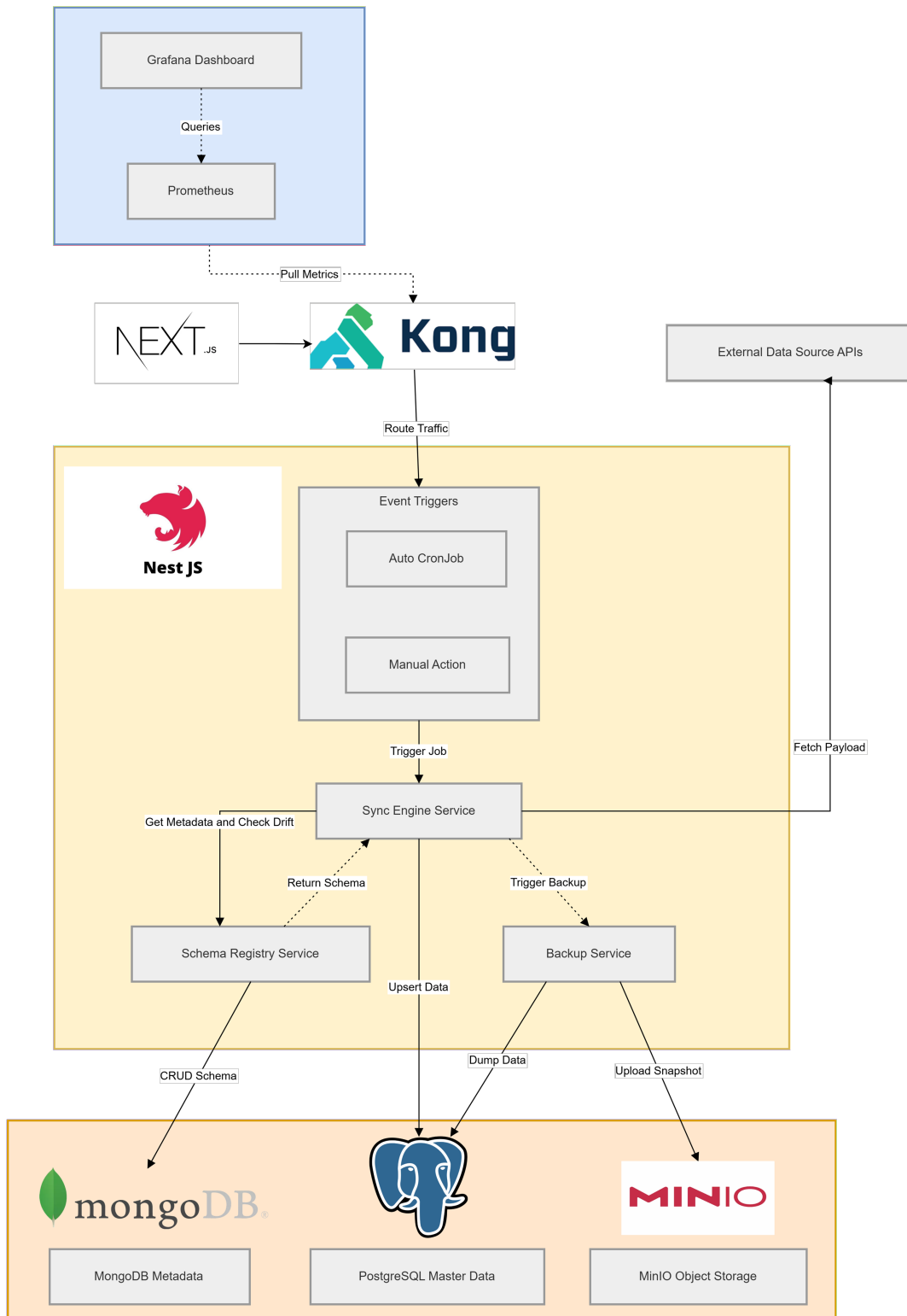
Hình 5.2: Tương tác giữa các module backend và với các thành phần bên ngoài
