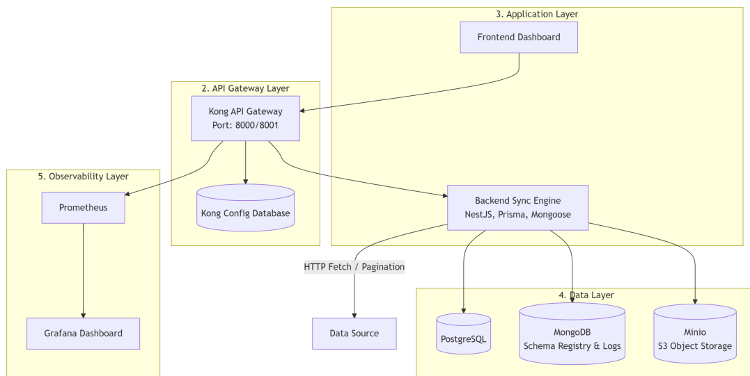
Hình 5.1: Sơ đồ kiến trúc tổng thể
