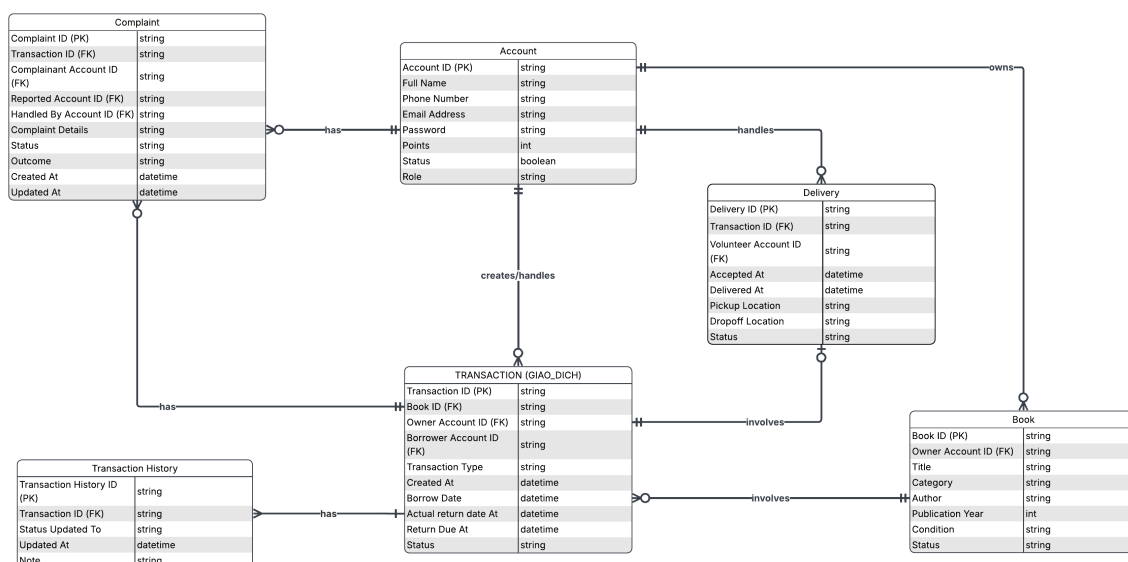
Figure 3: Mô hình thực thể liên kết của cơ sở dữ liệu hệ thống trao đổi sách
