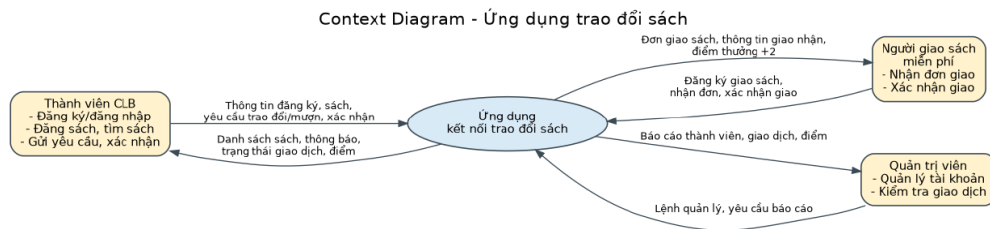
Figure 1: Biểu đồ ngữ cảnh của hệ thống kết nối thành viên trao đổi sách trong câu lạc bộ
