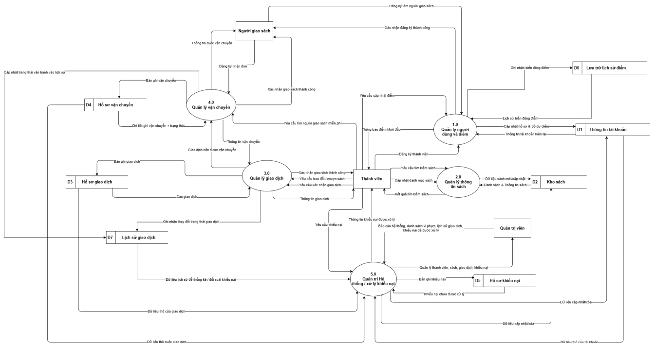
Figure 2: Biểu đồ luồng dữ liệu mức 0 của hệ thống trao đổi sách
