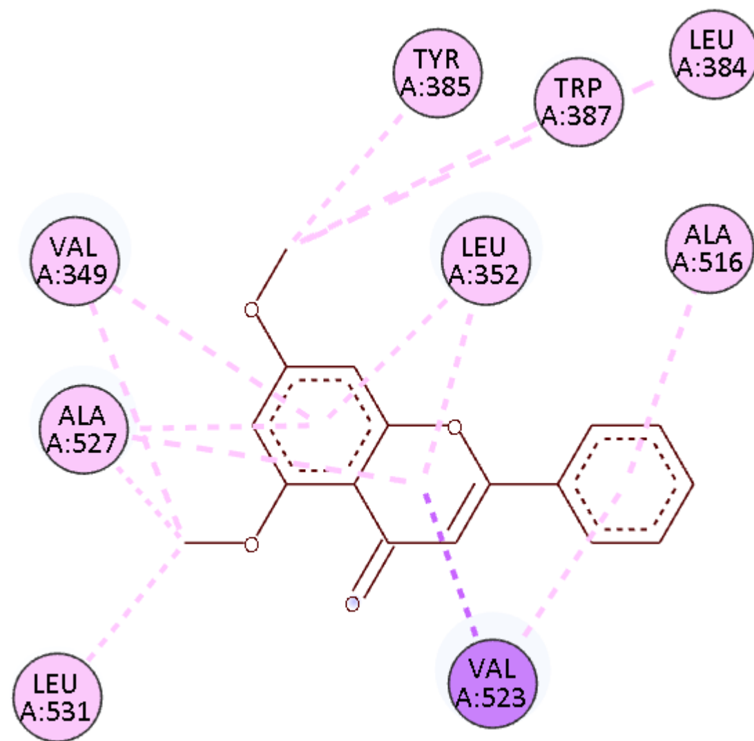
B) Ligand 15: 5,7-dimethoxyflavone
