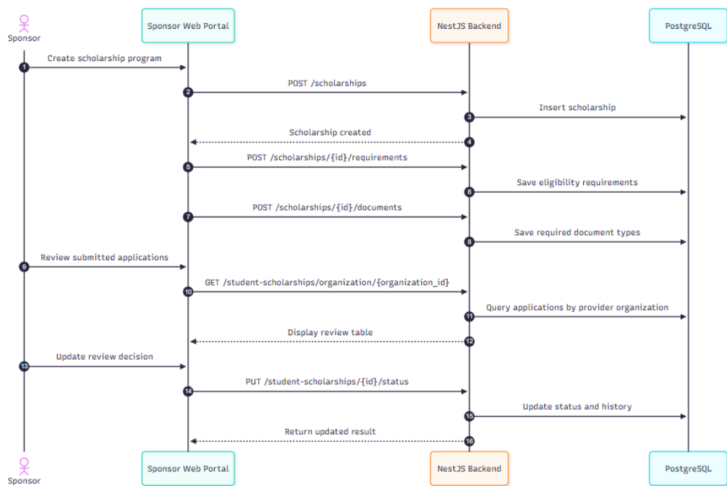
Hình 3.10: Sơ đồ luồng nhà tài trợ tạo, cấu hình và xét duyệt học bổng
