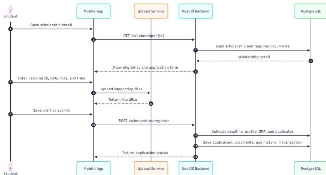
Hình 3.9: Sơ đồ luồng sinh viên xem, lưu nháp và nộp hồ sơ học bổng
