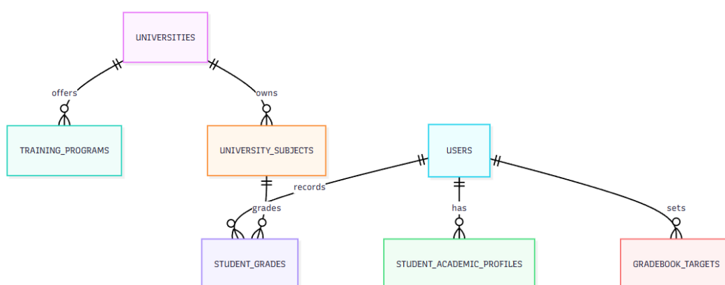
Hình 3.3: Sơ đồ ERD cho dữ liệu học thuật và bảng điểm sinh viên
