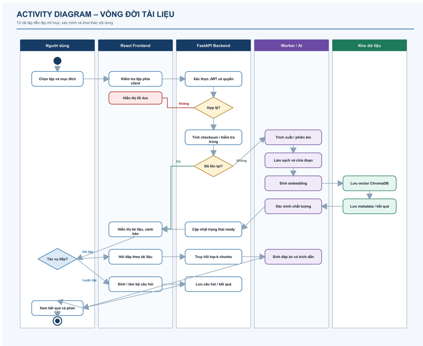
Hình 2. Activity Diagram vòng đời tài liệu và các hướng khai thác.
