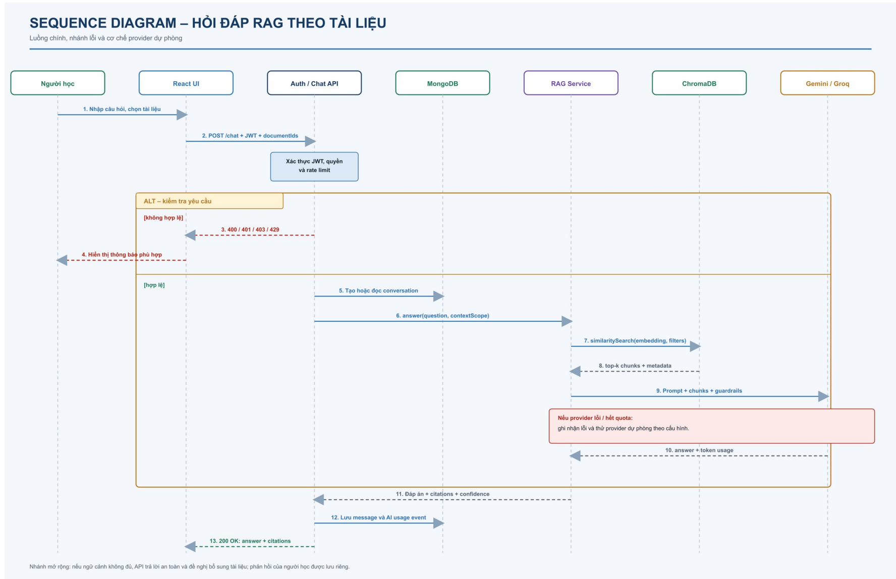
Hình 3. Sequence Diagram luồng hỏi đáp RAG theo tài liệu.
