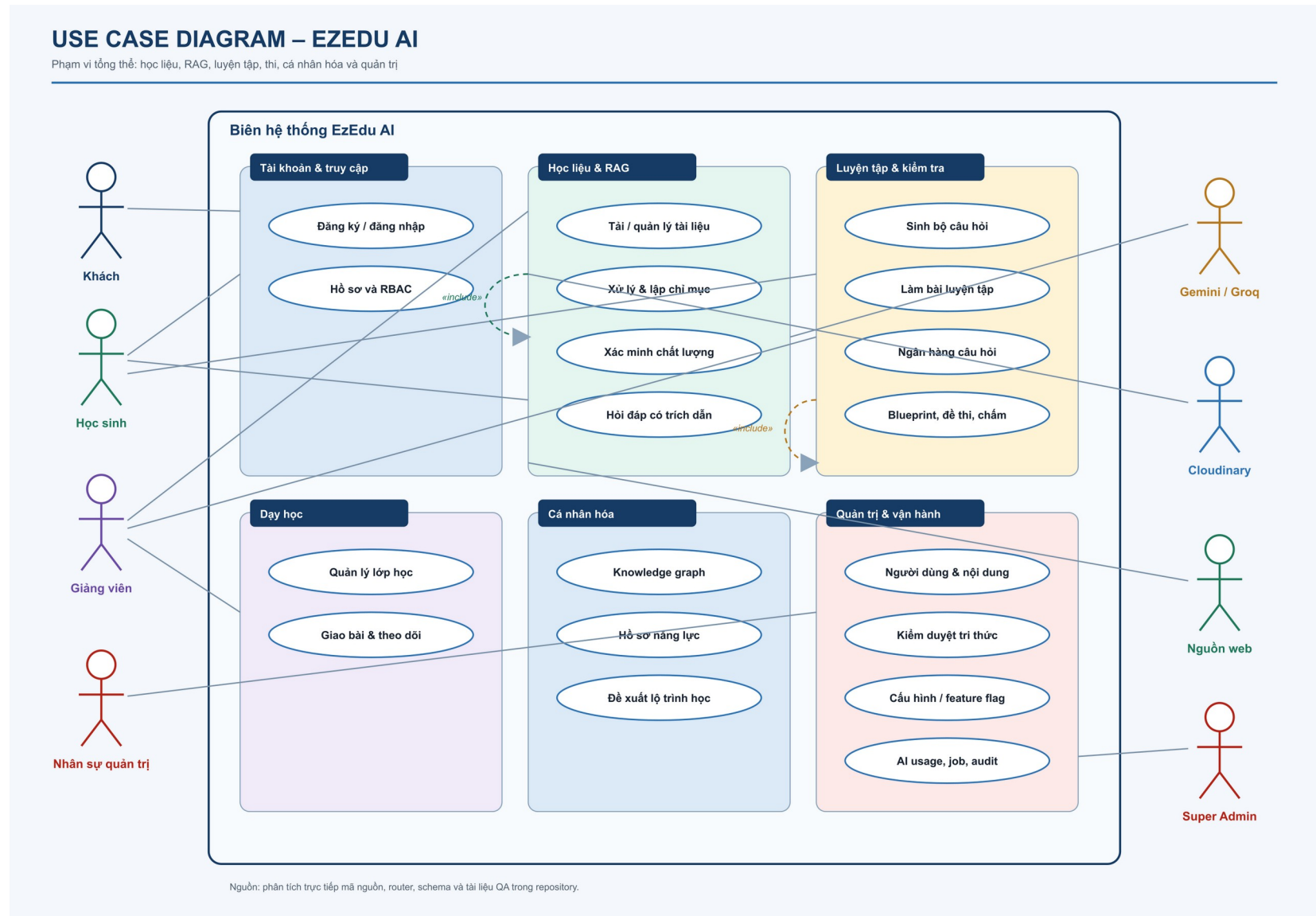
Hình 1. Use Case Diagram tổng thể của EzEdu AI.
