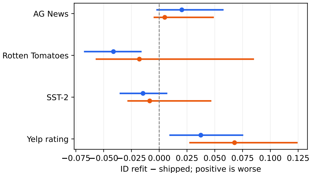
d1-omni — NLL
