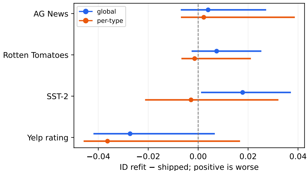
d1-3B — NLL
