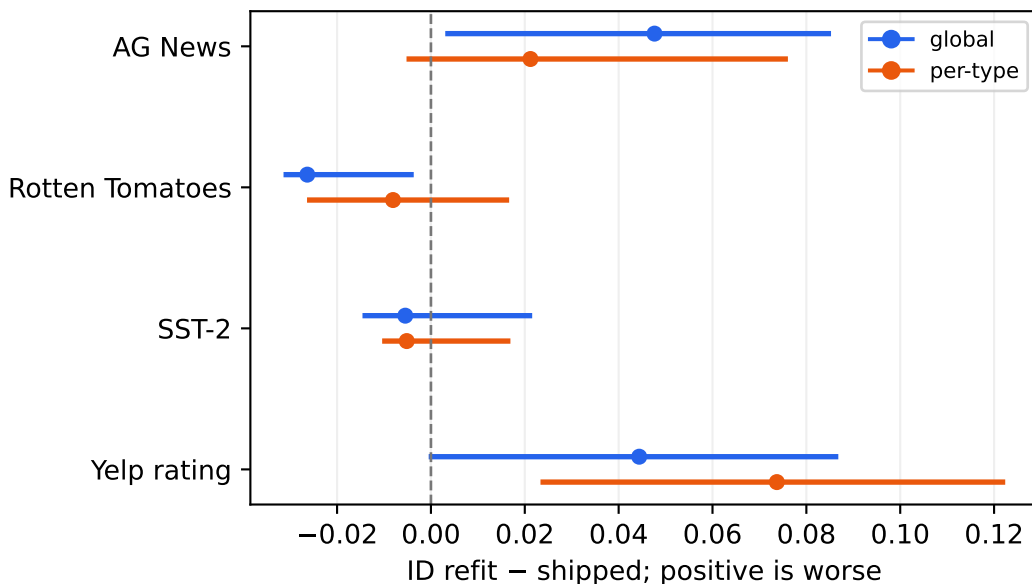
d1-omni — NLL
