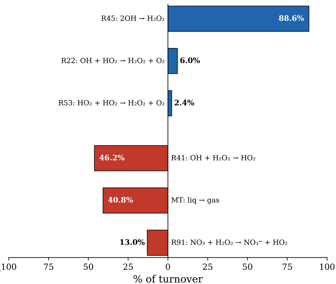
(d) \text{H}_2\text{O}_2
