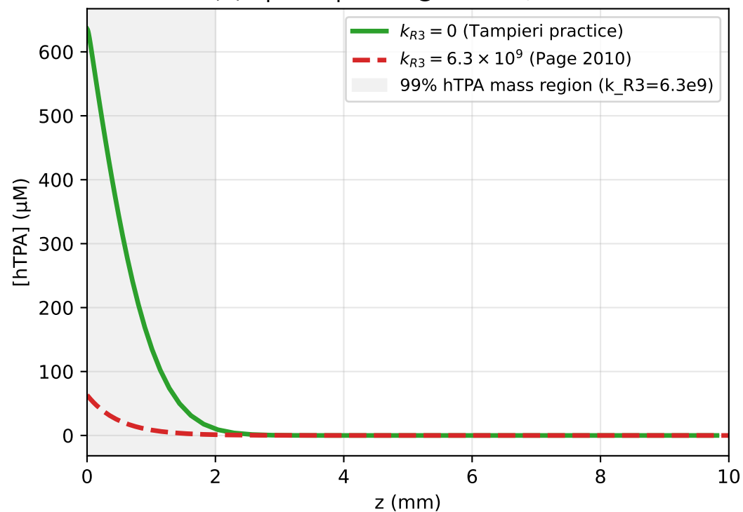
(d) Spatial profile @ t=600s, 3.2kV
