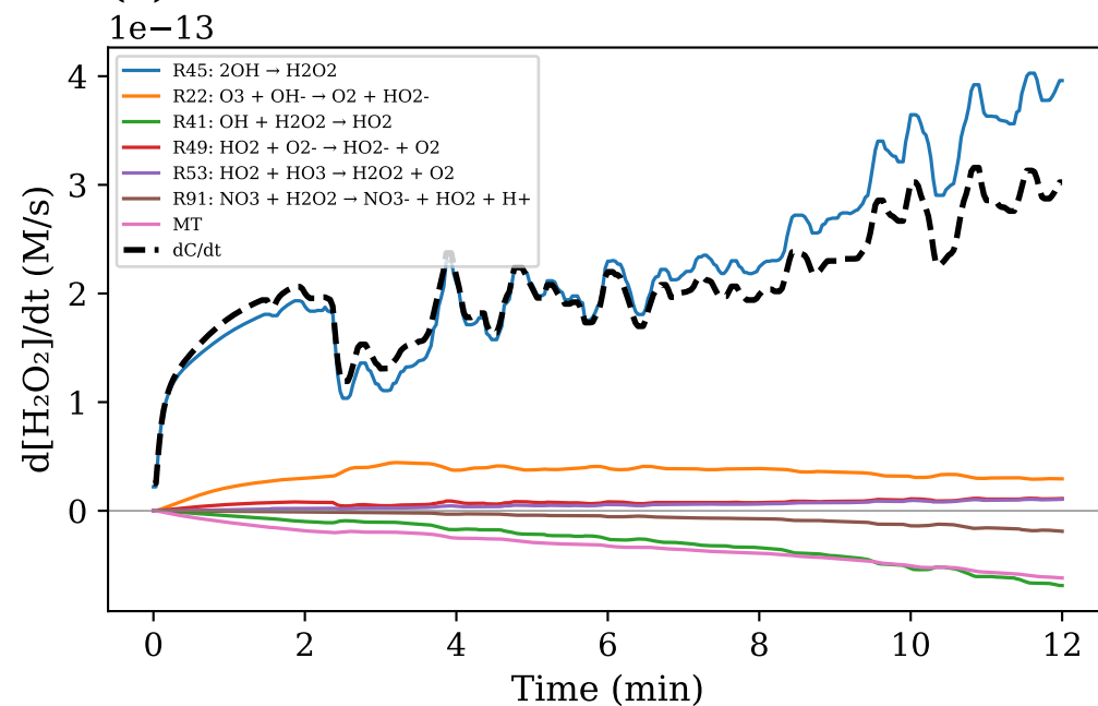
(d) H 2 O 2
