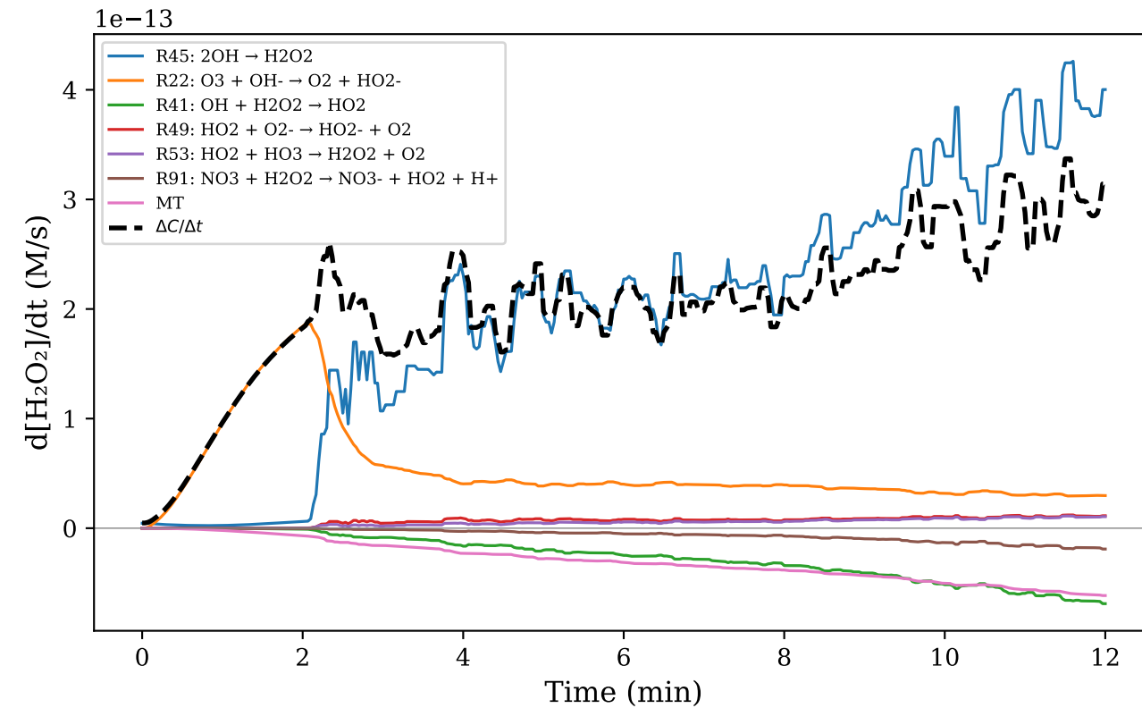
(d) \text{H}_2\text{O}_2
