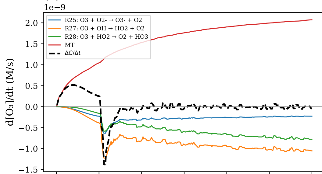
(d) \text{H}_2\text{O}_2
