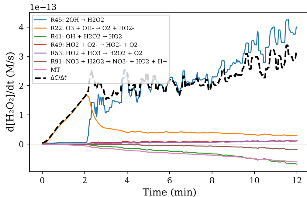
(d) \text{H}_2\text{O}_2
