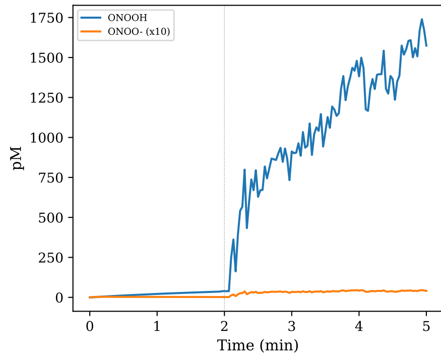
(d) ONOOH & ONOO - (surface)
