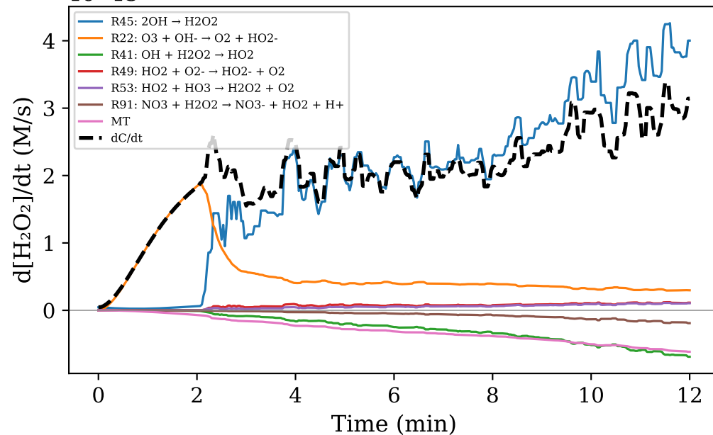
(d) \text{H}_2\text{O}_2
