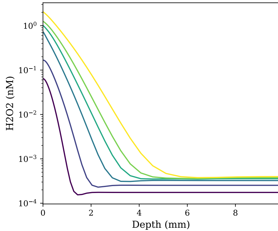
(d) H2O2
