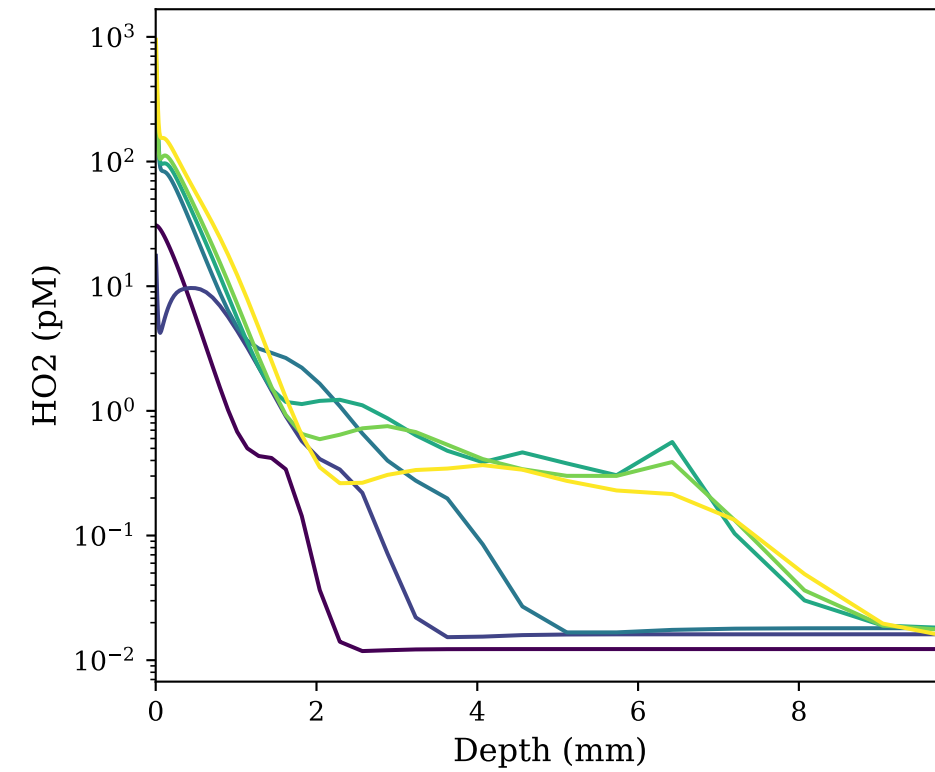
(f) HO2
