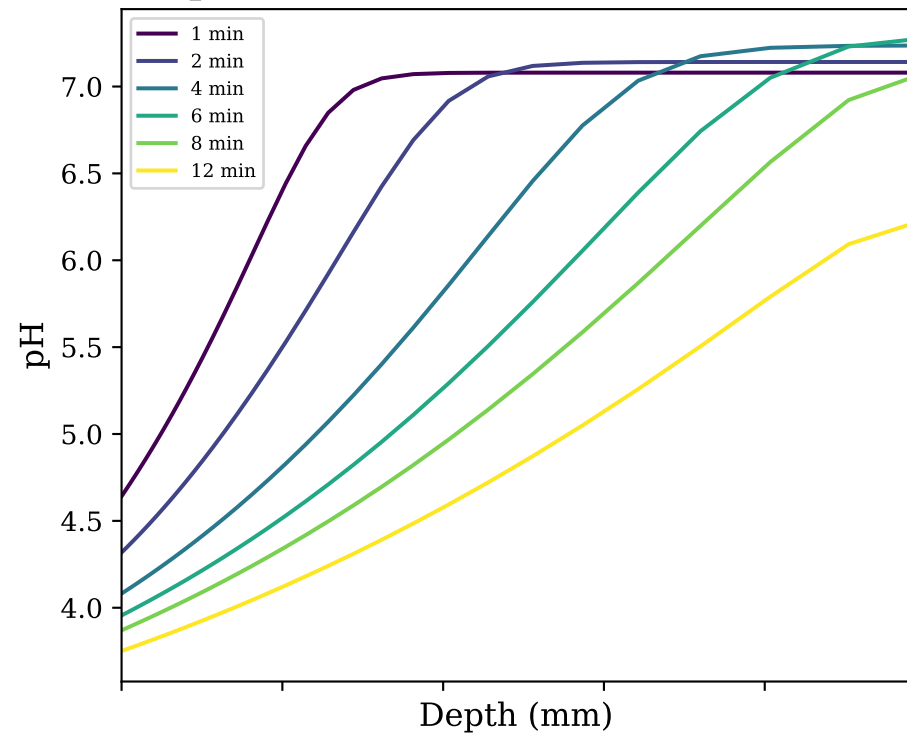
(d) H2O2
