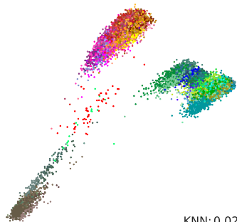
b PCA
