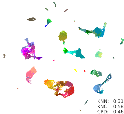
a Method: scVI (Latent Dim: 10)
