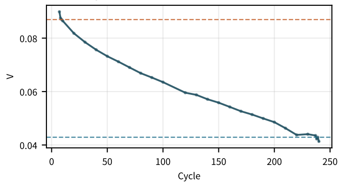
방전 플래토 \Delta V decreasing · -0.0317/100
