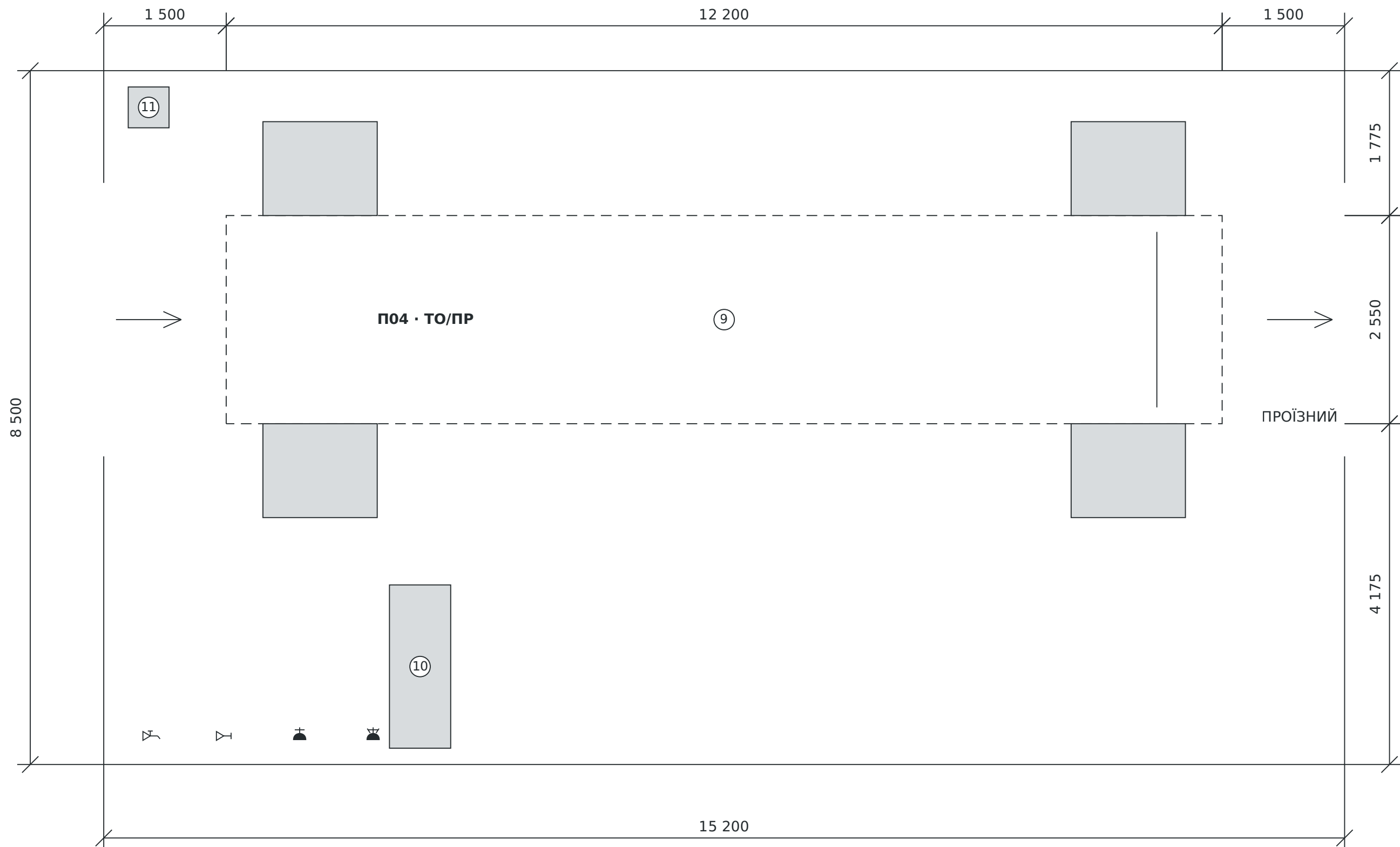
Рисунок А2.1 — Оснащений пост. Масштаб 1:50 за друку 100%.
