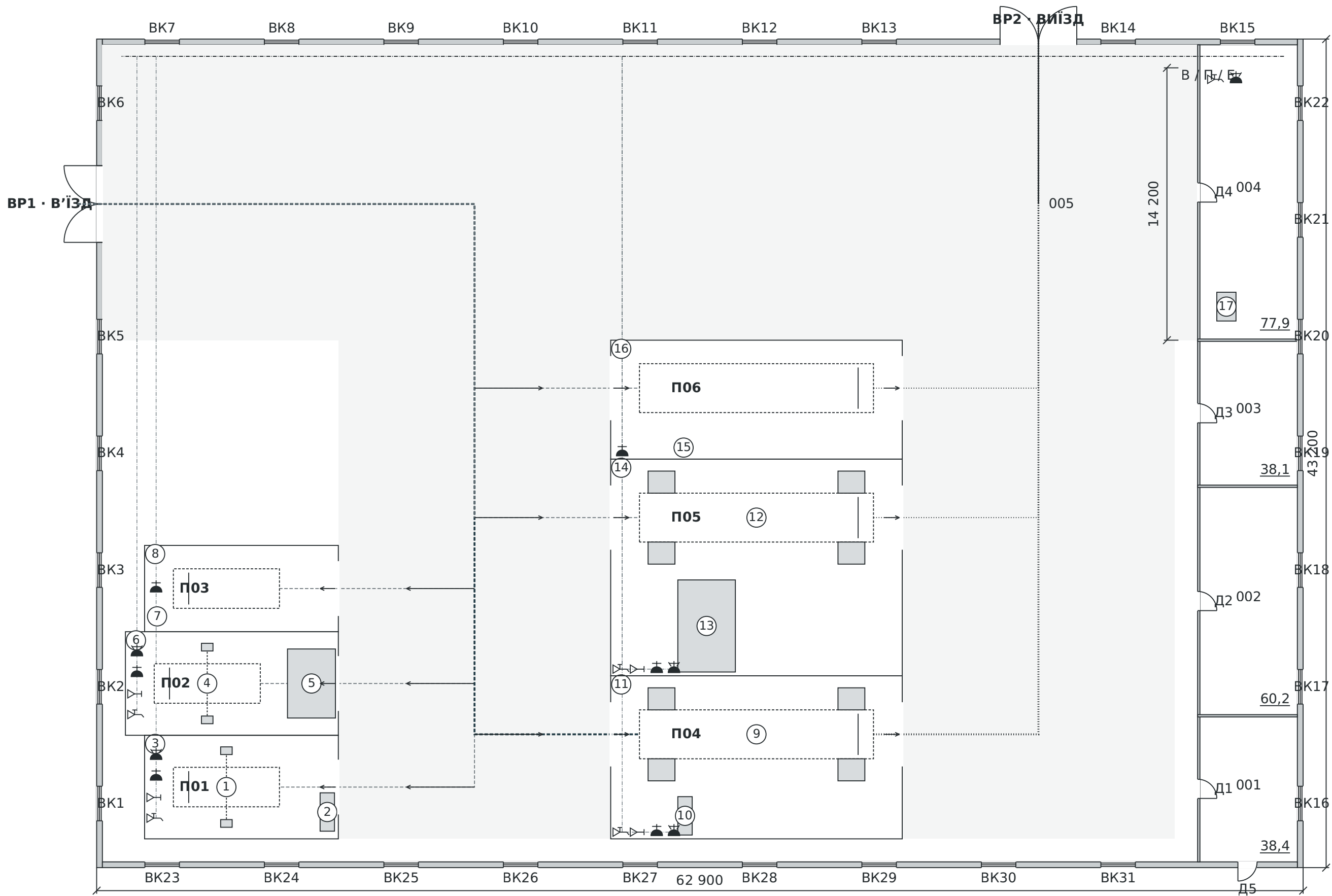
Рисунок А1.1 — План корпусу. Масштаб 1:200 за друку 100%.
