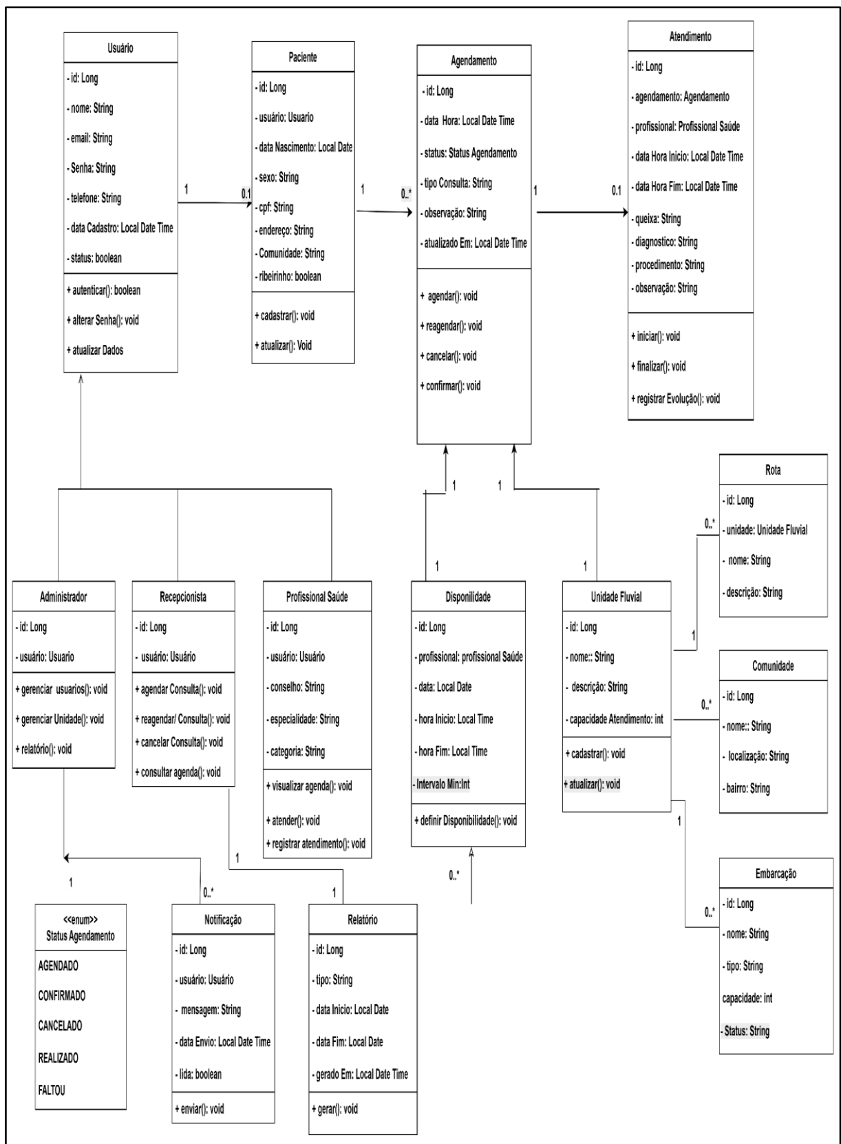
Figura: Diagrama de Classe.
