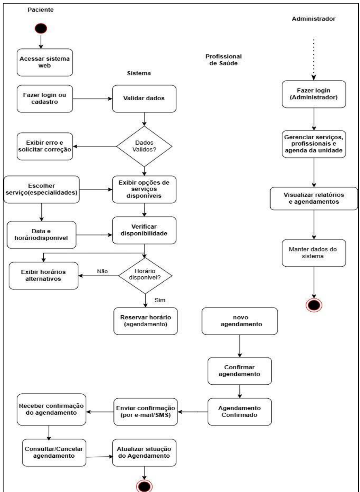
Figura 1. Diagrama de Atividade.
