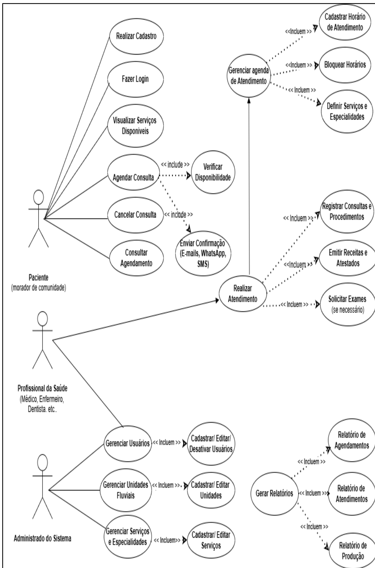
Figura: Diagrama de Caso de Uso.
