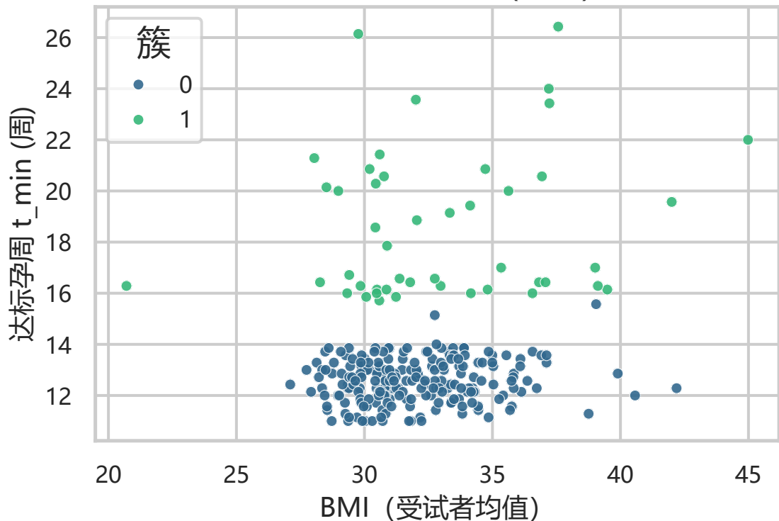
达标孕周 vs BMI (K=2)
