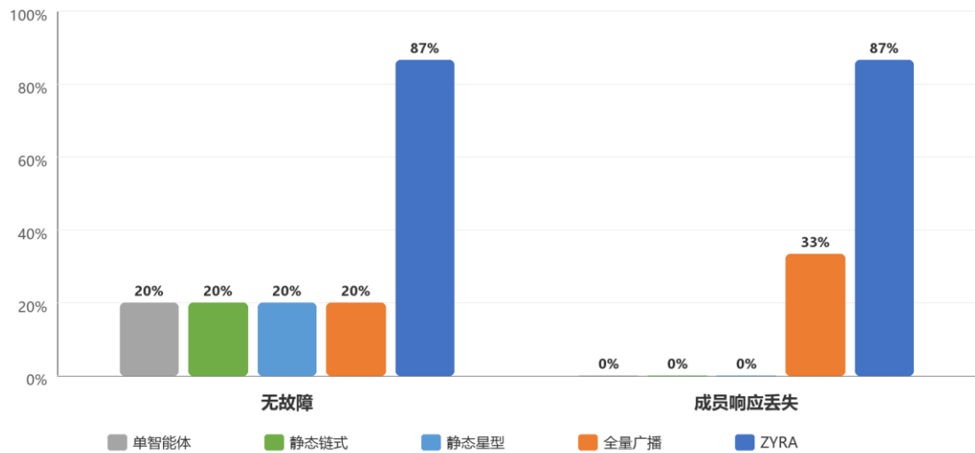
图 7 在线先导实验的严格任务成功率
