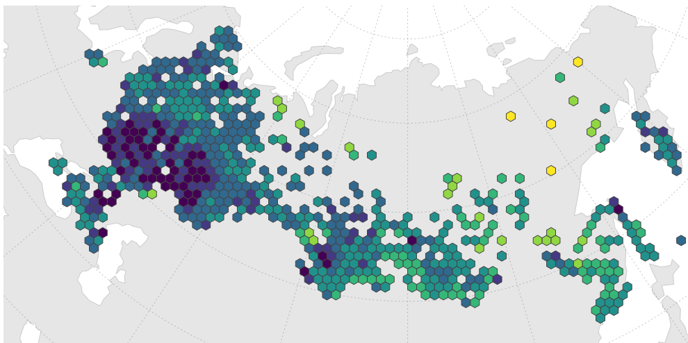
(b) FDC slope
