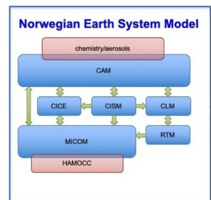
Illustration 2: Représentation des différentes composantes du modèle NorESM1
