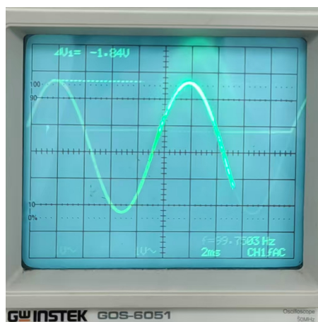
图 4: 测量时示波器显示图形
