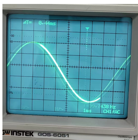
图 5: 测量时示波器显示图形
