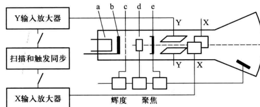
图 1: 示波器原理图
