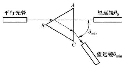
图 1: 最小偏向角原理
