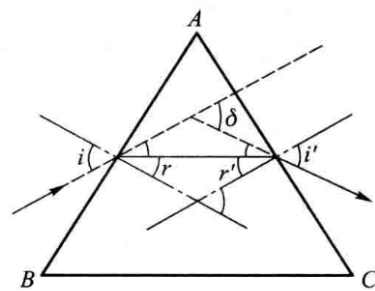
图 2: 折射率测量光路图
