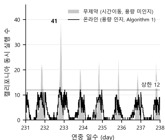
그림 9. 시간 이동 전후 캘리포니아의 동시 실행 수 — 연중 한 주(day 231–238)의 예시다. 회색 영역은 용량을 보지 않은 시간 이동, 검은 선은 온라인 용량 인지(Algorithm 1)이며, 점선은 유효 상한 12다. 온라인의 연중 최대 17건은 이 주가 아닌 다른 주에서 난다.
