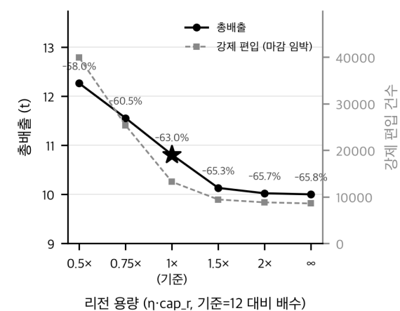
용량 6→∞로 늘리면 총배출은 12.26~10.00 t(58.0~65.8%)로, 강제 편입은 39,903~8,572건으로 함께 준다. 모든 구간 마감위반 0.
