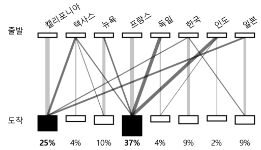
그림 5. 공간 이동이 만든 리전 간 흐름 — 1년치 146,000건의 실제 배정이다. 옮긴 물량의 91%를 차지하는 흐름 10개만 그렸다. 회색 세로선은 홈에 남은 몫이고, 20% 넘게 받은 두 리전을 검게 칠했다. 8×8 배정 행렬 전체는 추가자료에 있다.
