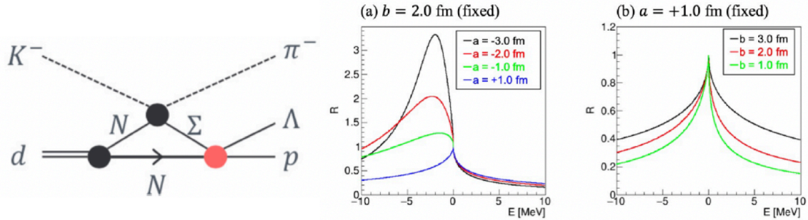
図 4: J-PARC E90 実験における \Sigma N カusp生成の反応ダイアグラム（左）と、 \Sigma N 散乱長の実部 a ・虚部 b を変化させた場合の質量スペクトル ( E = M - M_N - M_\Sigma ) の理論的な形状変化デモンストレーション（右）。散乱長の違いが極めて高い感度でスペクトル形状に反映される。
