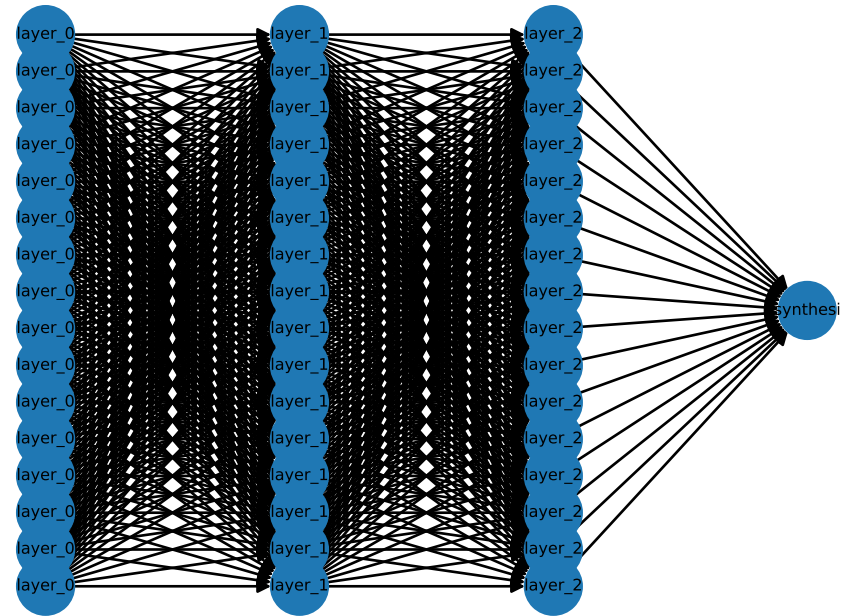
mesh_stress_moa
