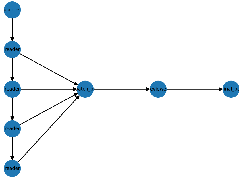
long_context_swe_stress
