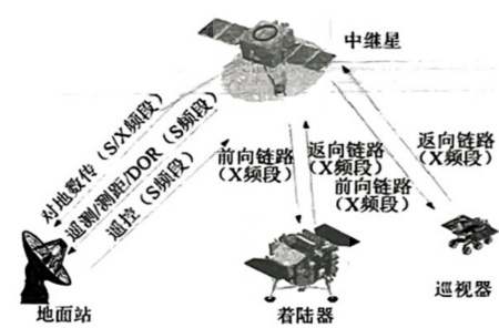
图 1 探月工程中的通信原理图
