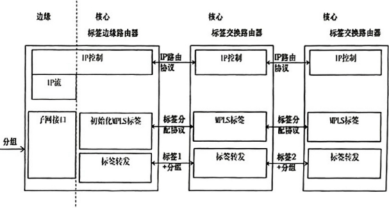
图 2 MPLS 网络原理（功能）图
