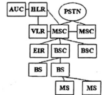
蜂窝移动通信系统基本结构
