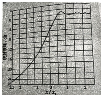
图2 绕射损耗与菲涅尔余隙之间的关系
