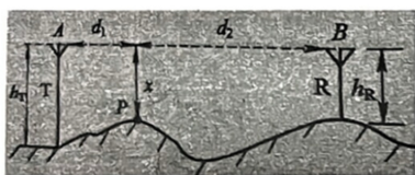
图1 两天线间传输路径
