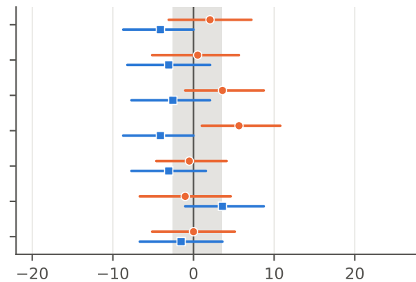
Gemma-2-9B: sycophancy, TruthfulQA
