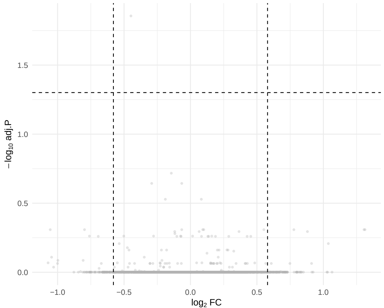
Volcano (limma): HY vs DO
