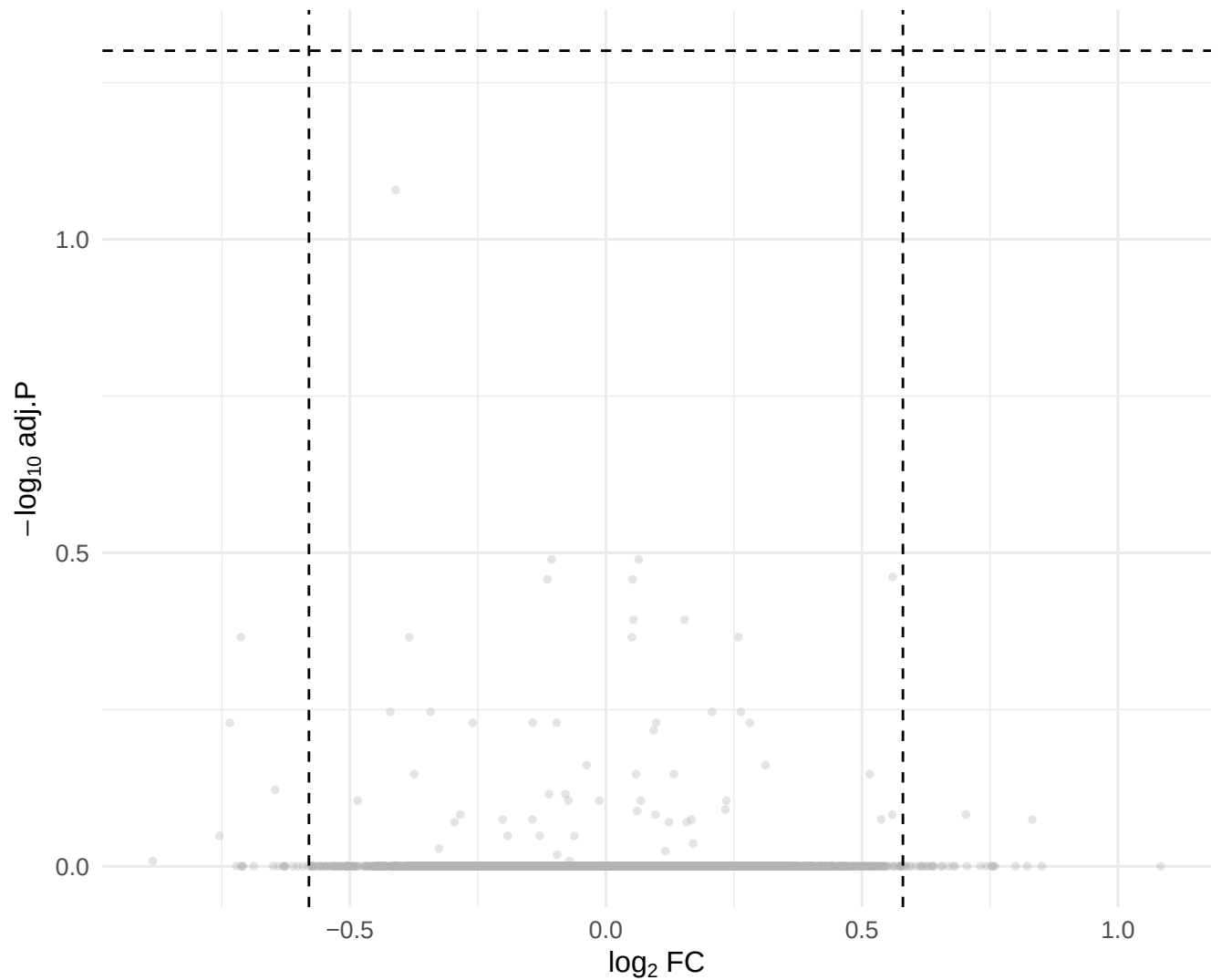
Volcano (limma): HO vs HY
