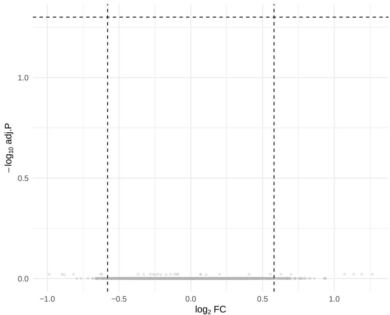
Volcano (limma): HO vs DO
