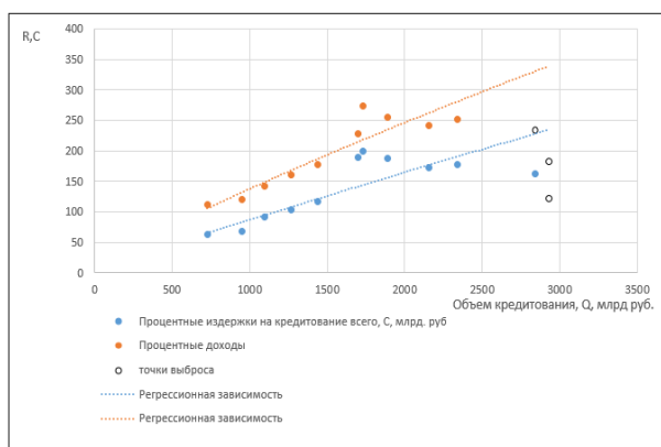
Рис. 1. Функции процентных доходов и расходов: а – для Сбербанка, б – для ВТБ, в – для Альфабанка, г – для Газпромбанка, д – для Россельхозбанка, е – для ТБанка
