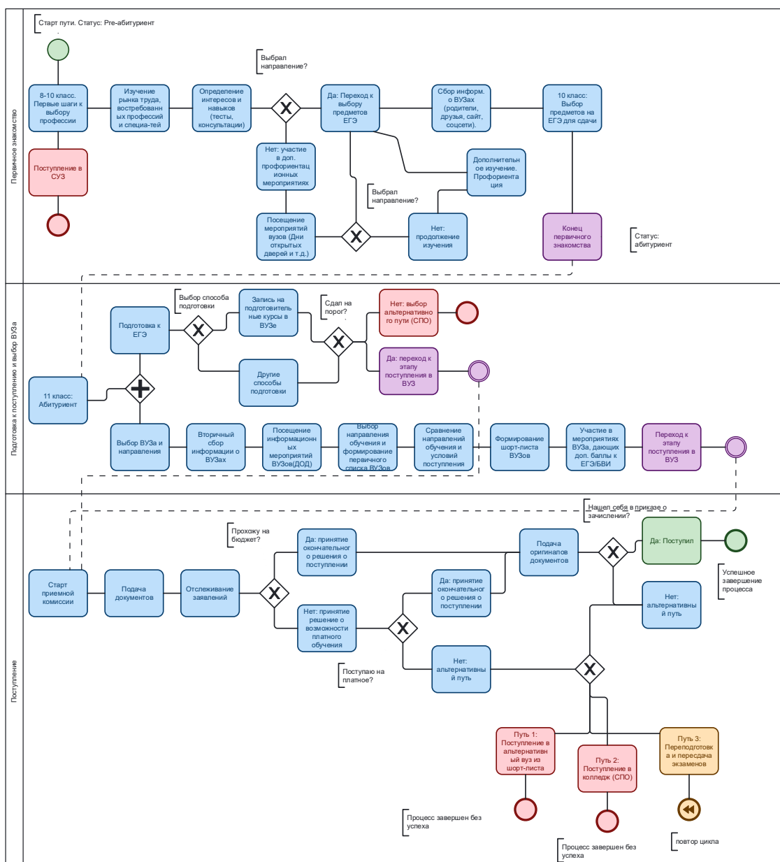
Рис. 2. Нотация BPMN для описания пути абитуриента
