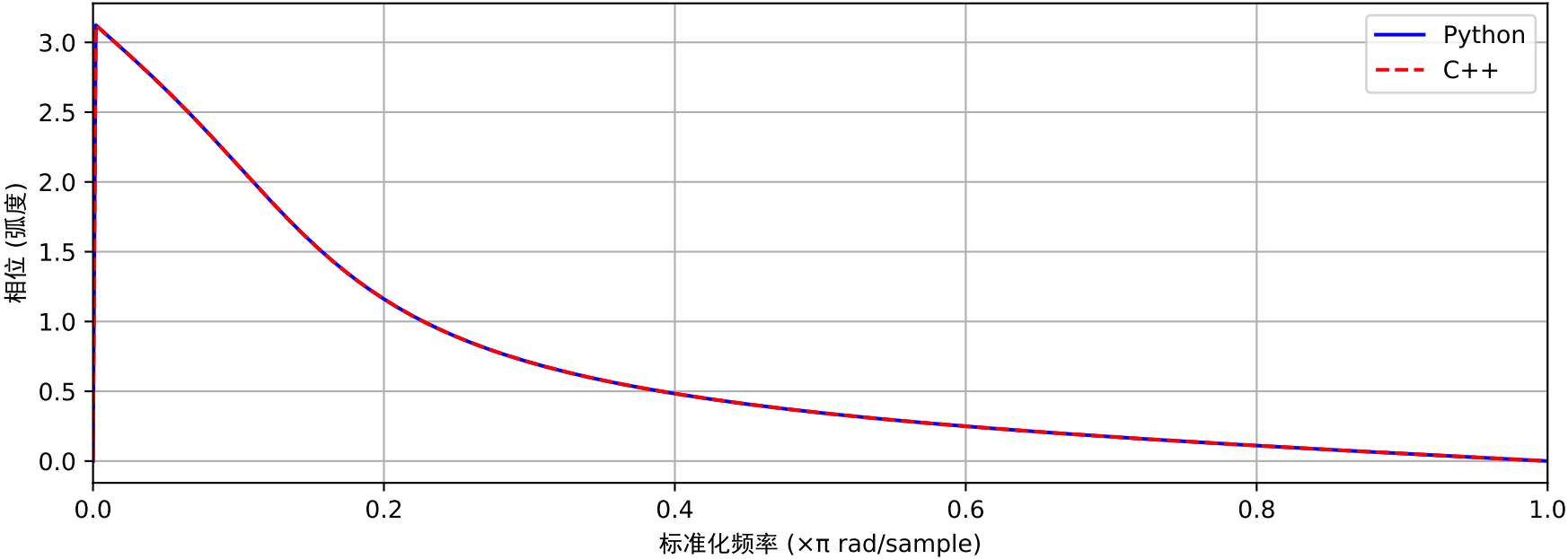
相位响应
