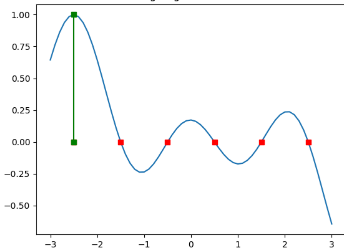
lagrange function 0
