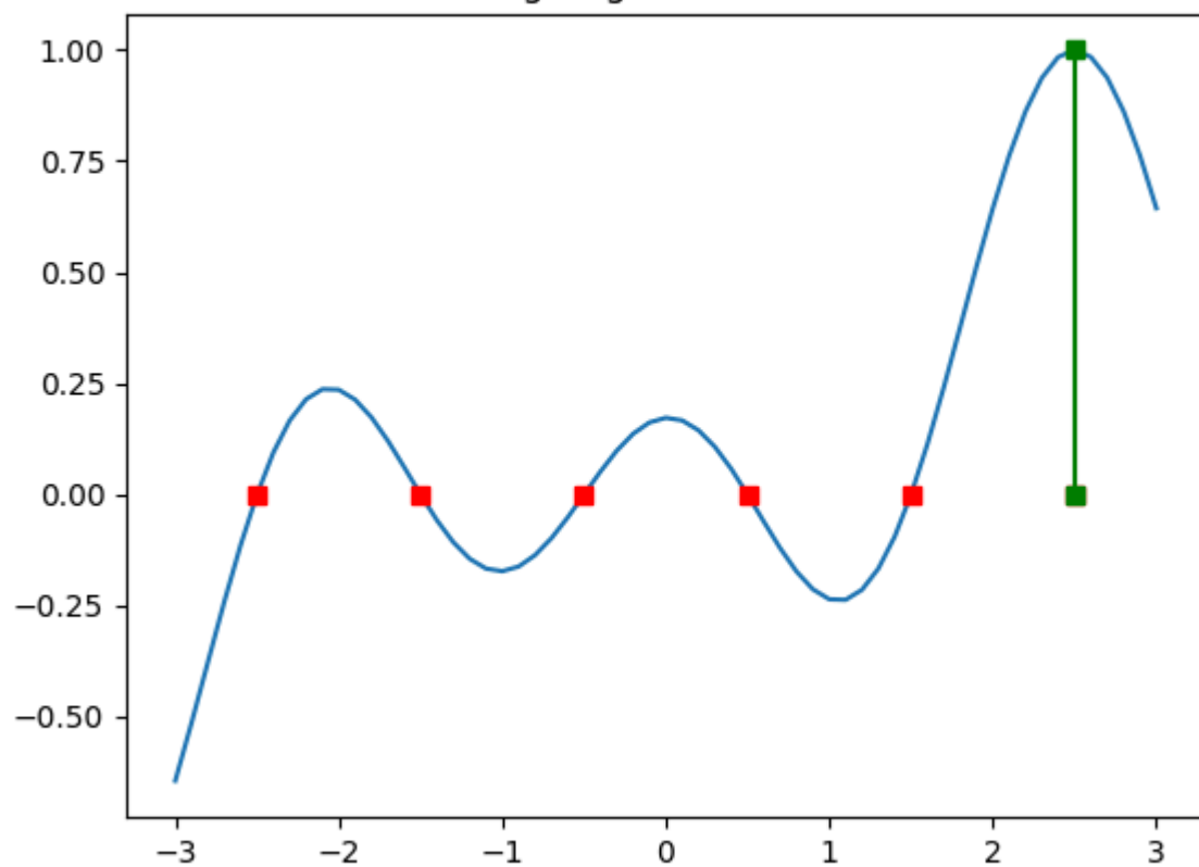
lagrange function 5
