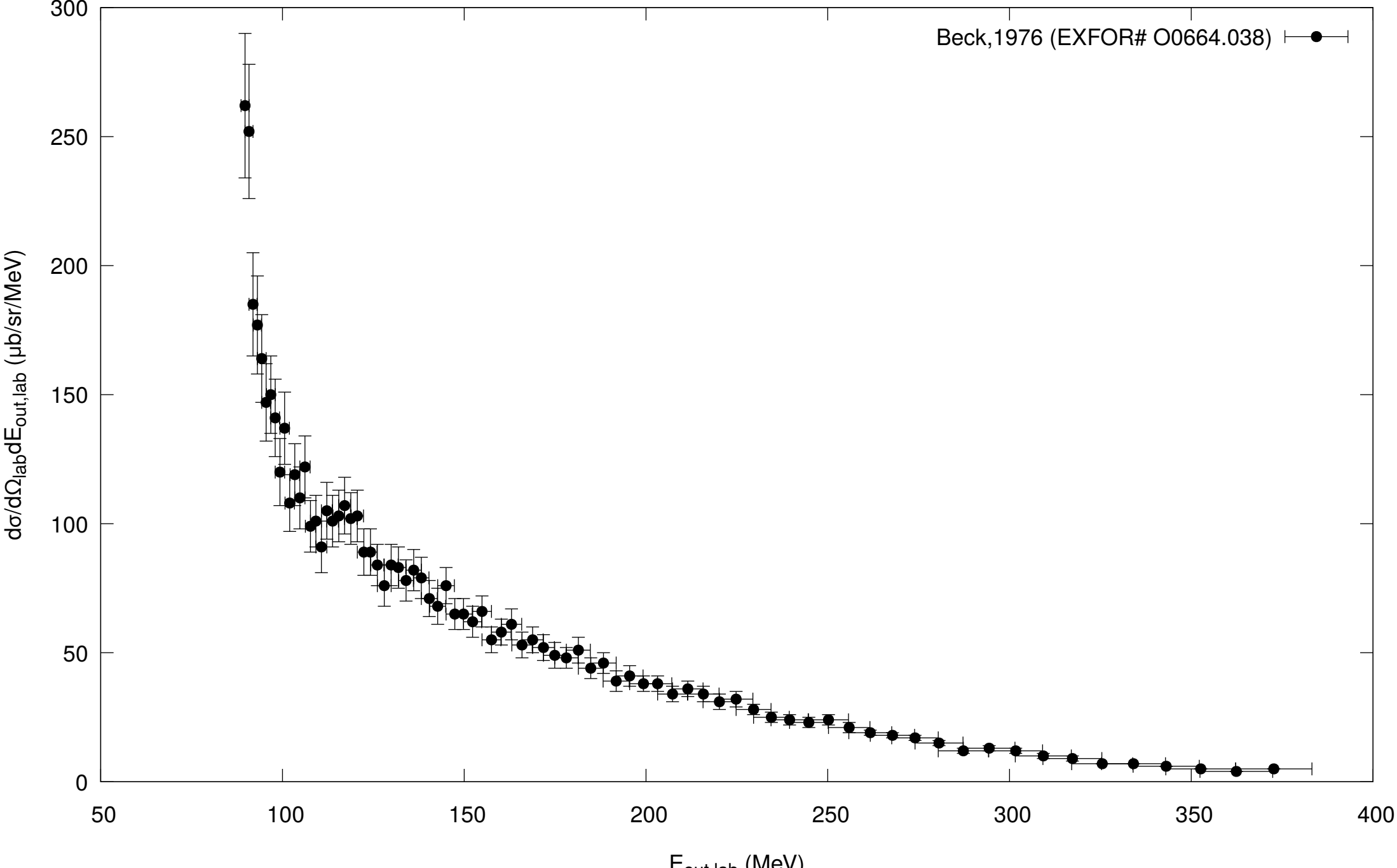
Cu(p,d+x), E_{\text{inc}}=558 MeV, \theta_{\text{lab}}=40 deg
