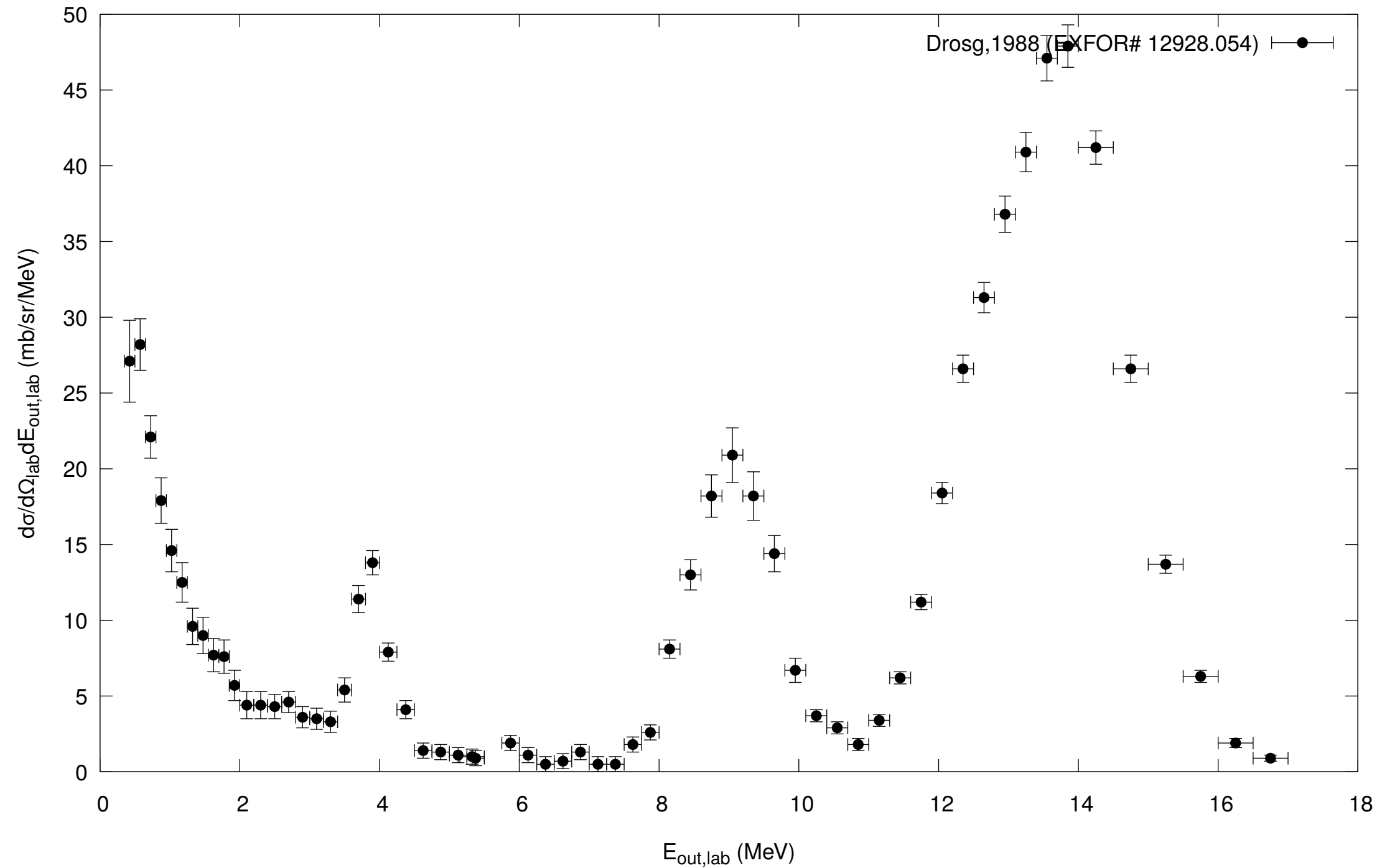
C(n,n+x), E_{\text{inc}}=14.1 MeV, \theta_{\text{lab}}=40 deg
