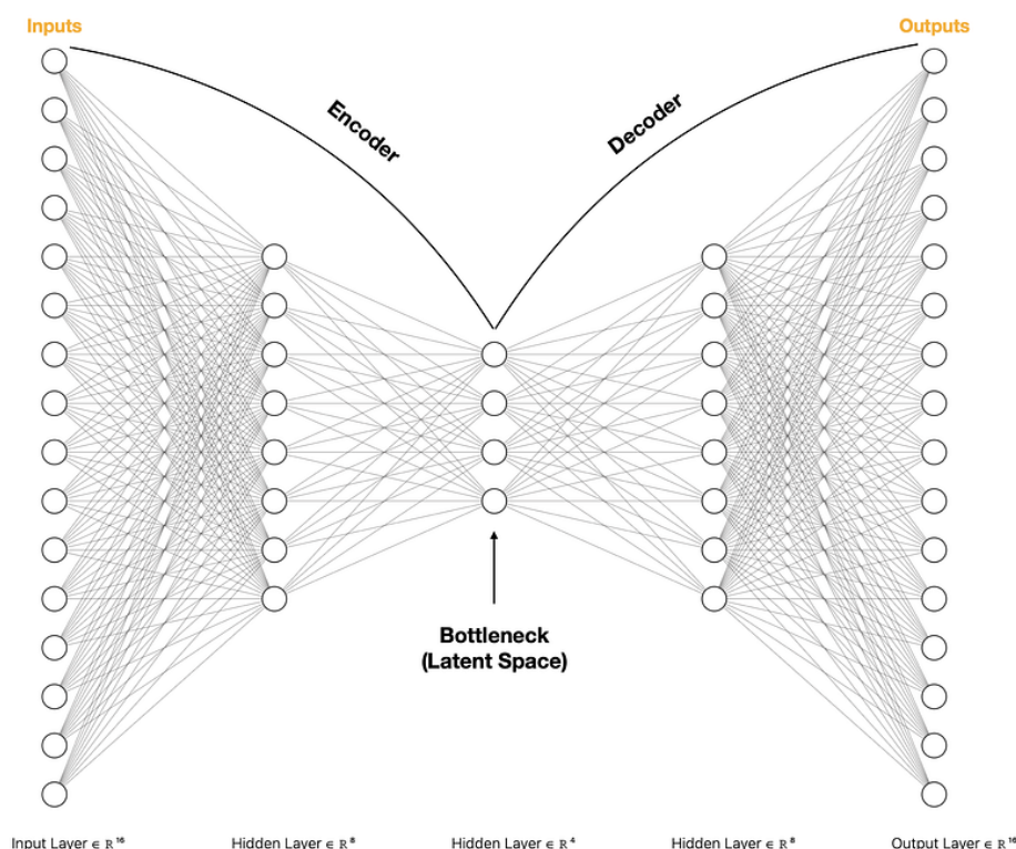
Рисунок 1.1 – Пример структуры автоэнкодера [1]
