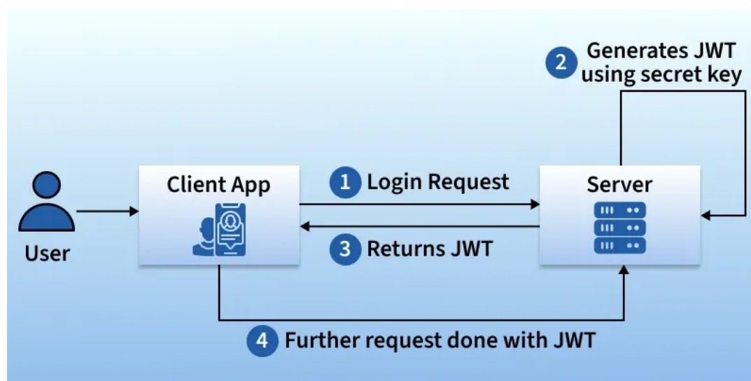
Рисунок 2.1 – Схема создания и использования аутентификационного токена [5]
