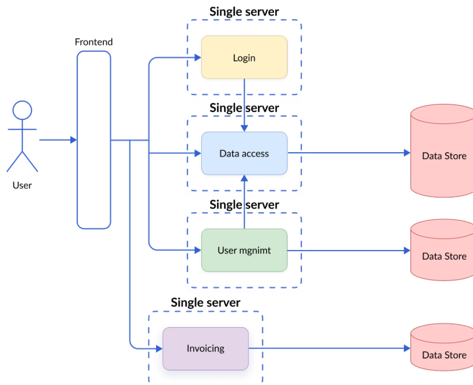
Рисунок 2.6 – Много микросервисов [4]
