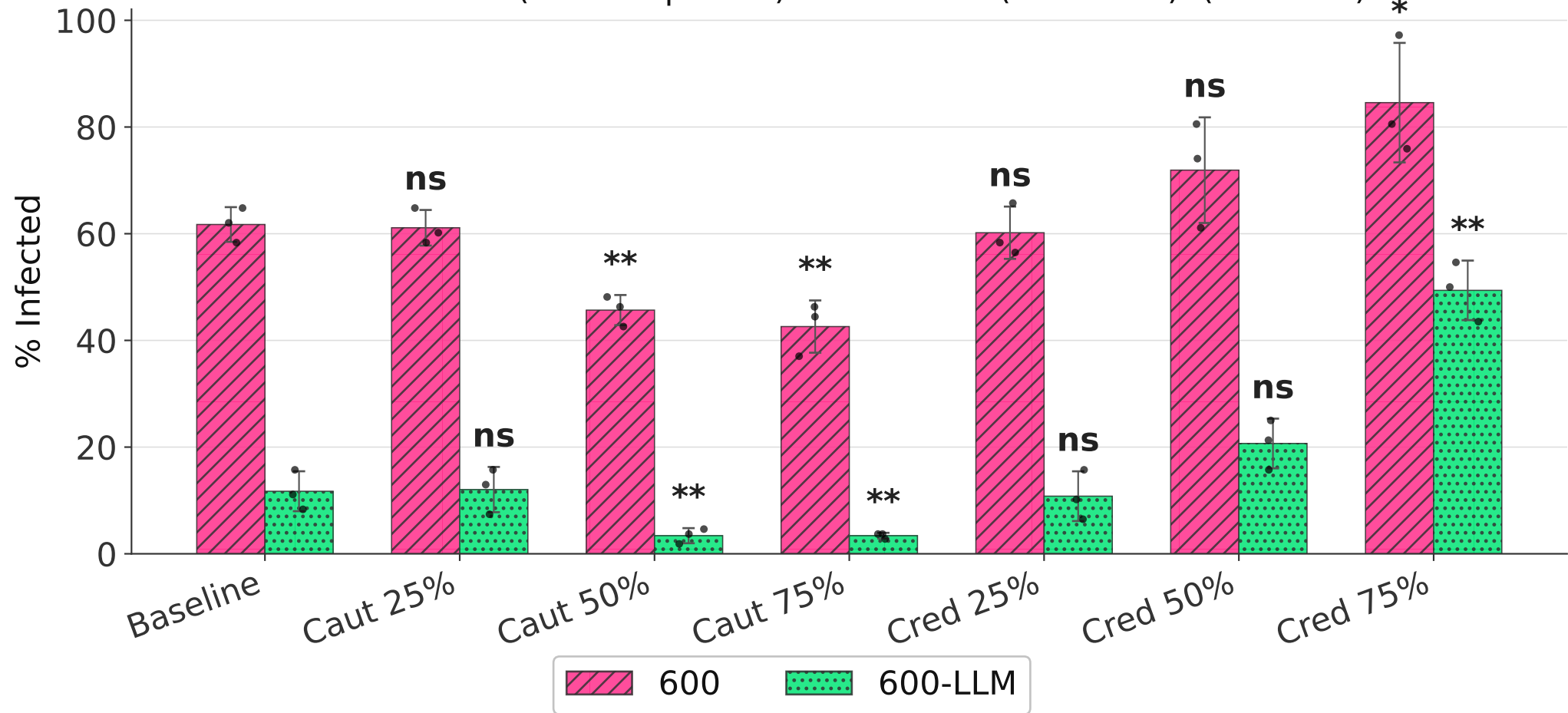
% Infected (of susceptibles) - Thread A (108 susc.) (absolute)
