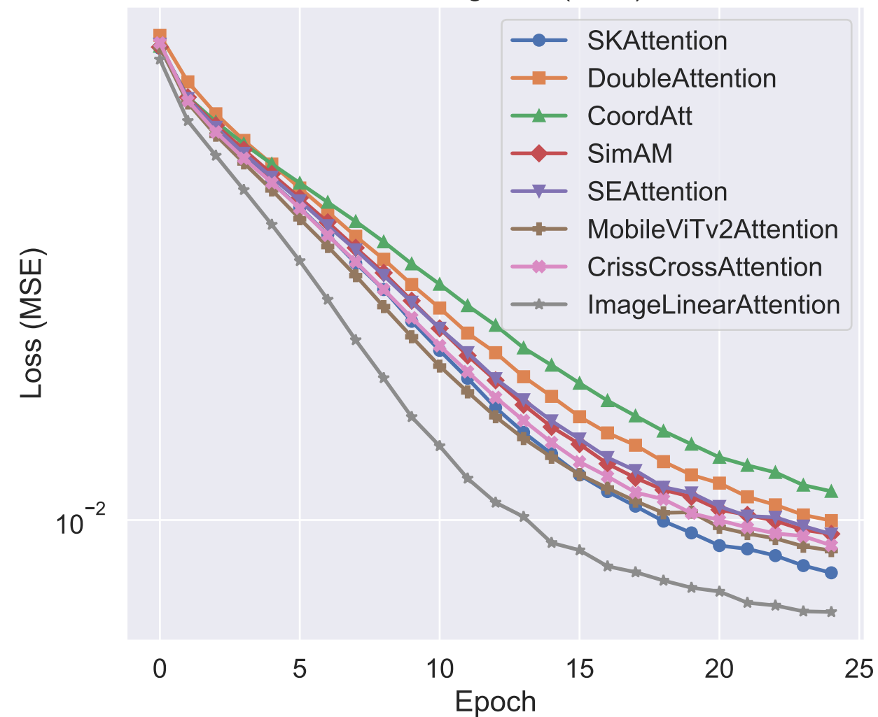
Finetuning Loss (MSE)
