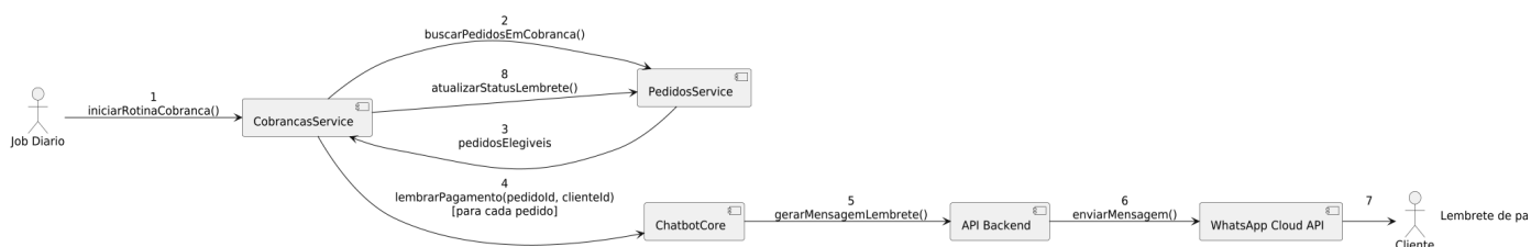
Figura 24 - Diagrama de Comunicação: Rotina de Cobrança (UC10 + regra)
