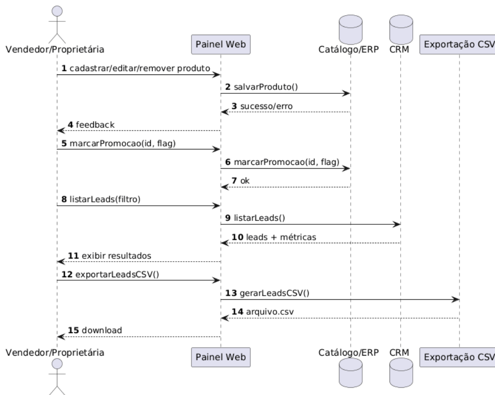
Figura 19 – Diagrama de sequência do sistema para o caso de uso C04.
