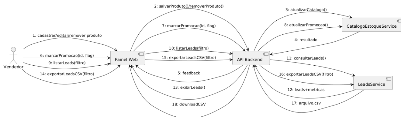
Figura 25 - Diagrama de Comunicação: Manter Catálogo e Leads (UC07-UC10)
