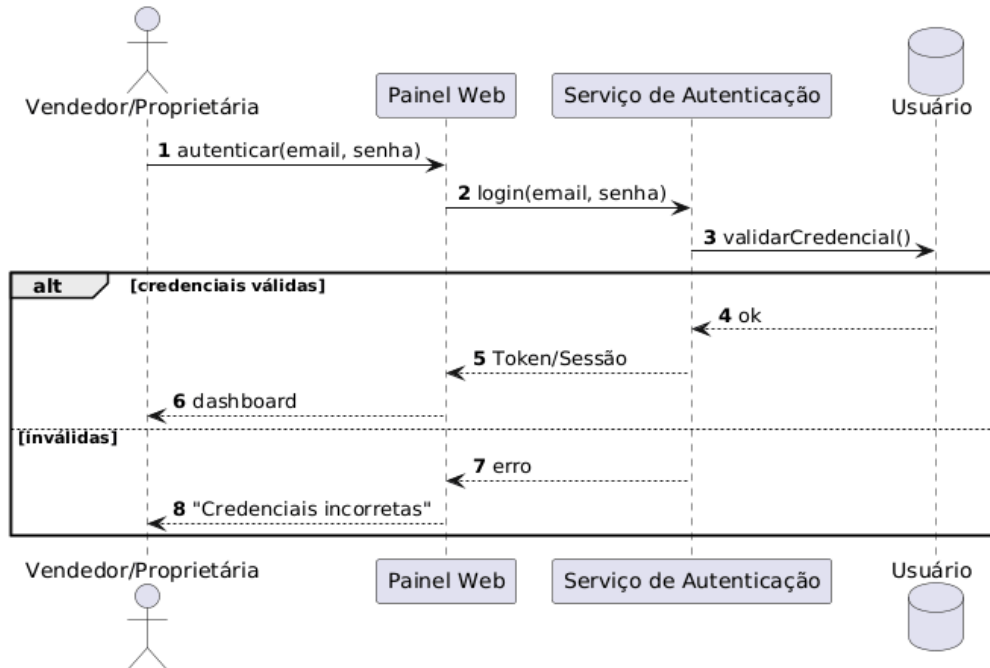
Figura 18 – Diagrama de sequência do sistema para o caso de uso C03.
