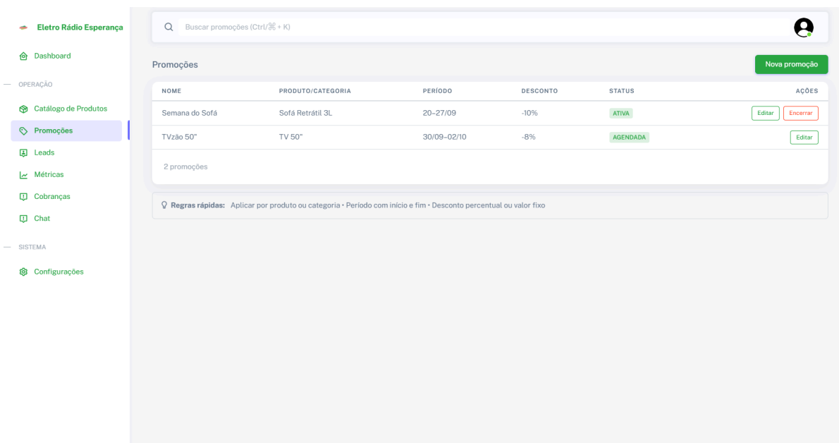
Figura 36 – Promoções cadastradas
