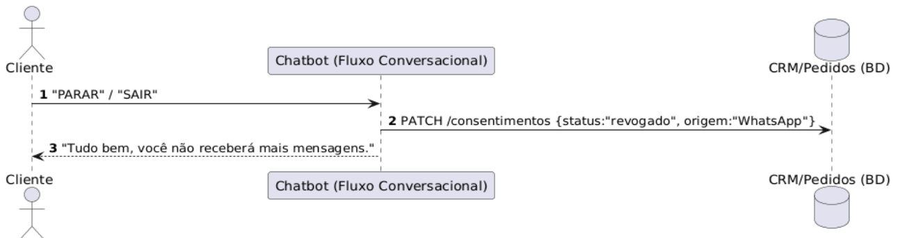
Figura 9 – DSS 5: Opt-out
