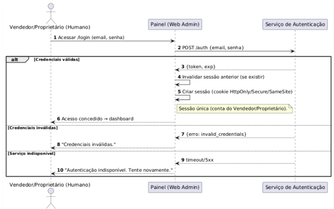
Figura 10 – DSS: Autenticação do Painel
