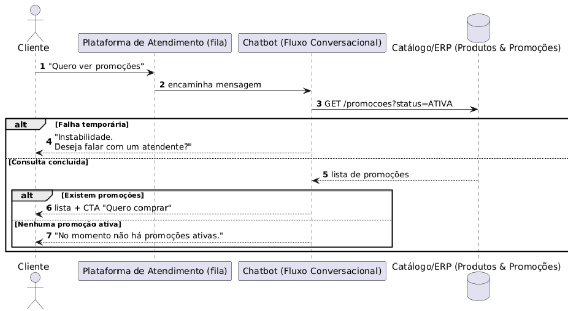
Figura 16 – Diagrama de sequência do sistema para o caso de uso C01.
