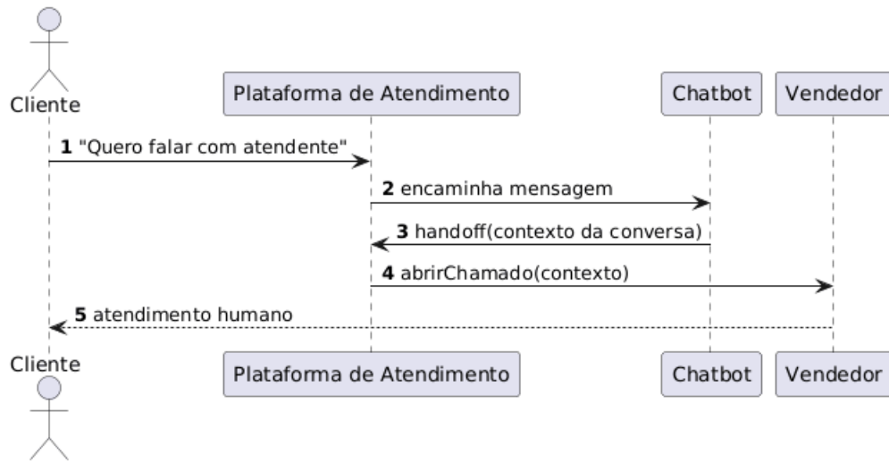
Figura 17 – Diagrama de sequência do sistema para o caso de uso C02.
