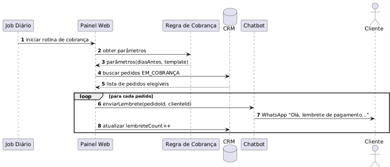
Figura 20 – Diagrama de sequência do sistema para o caso de uso C05.
