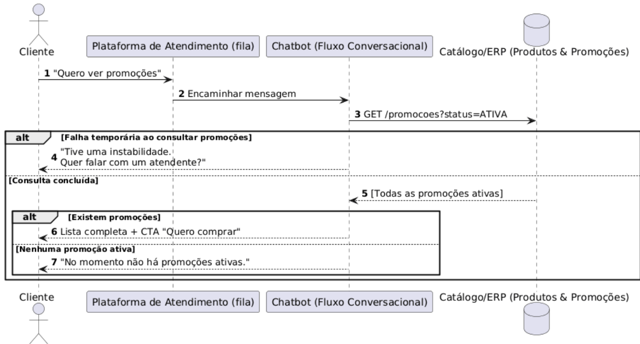
Figura 6 – DSS 2: Consultar Promoções
