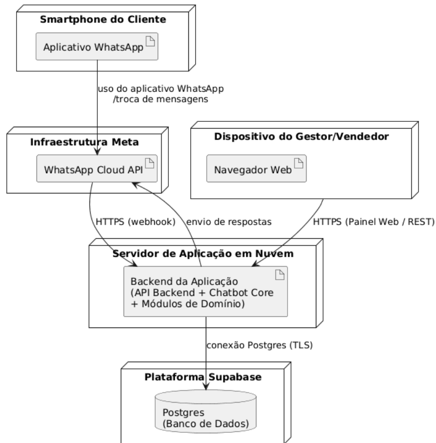
Figura 29 – Diagrama de Implantação
