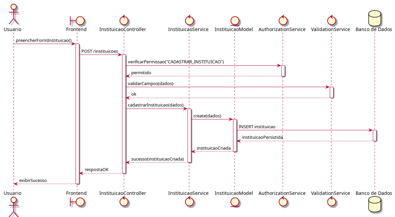
Figura 26 – Diagrama de Sequência: Cadastrar Instituição
