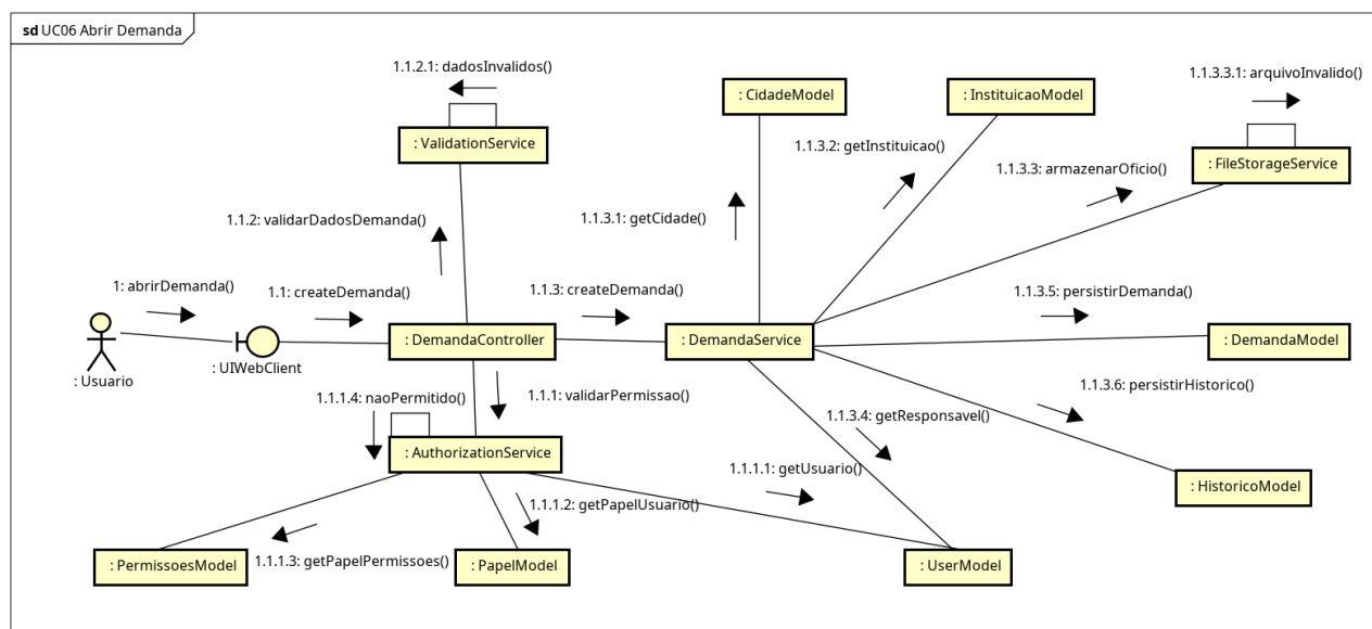
Figura 64 – Diagrama de Comunicação: Abrir Demanda
