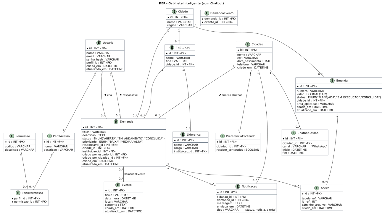
Figura 123 – Diagrama de Entidade e Relacionamento
