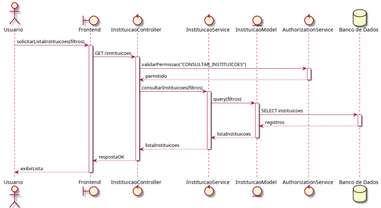
Figura 27 – Diagrama de Sequência: Consultar Instituição
