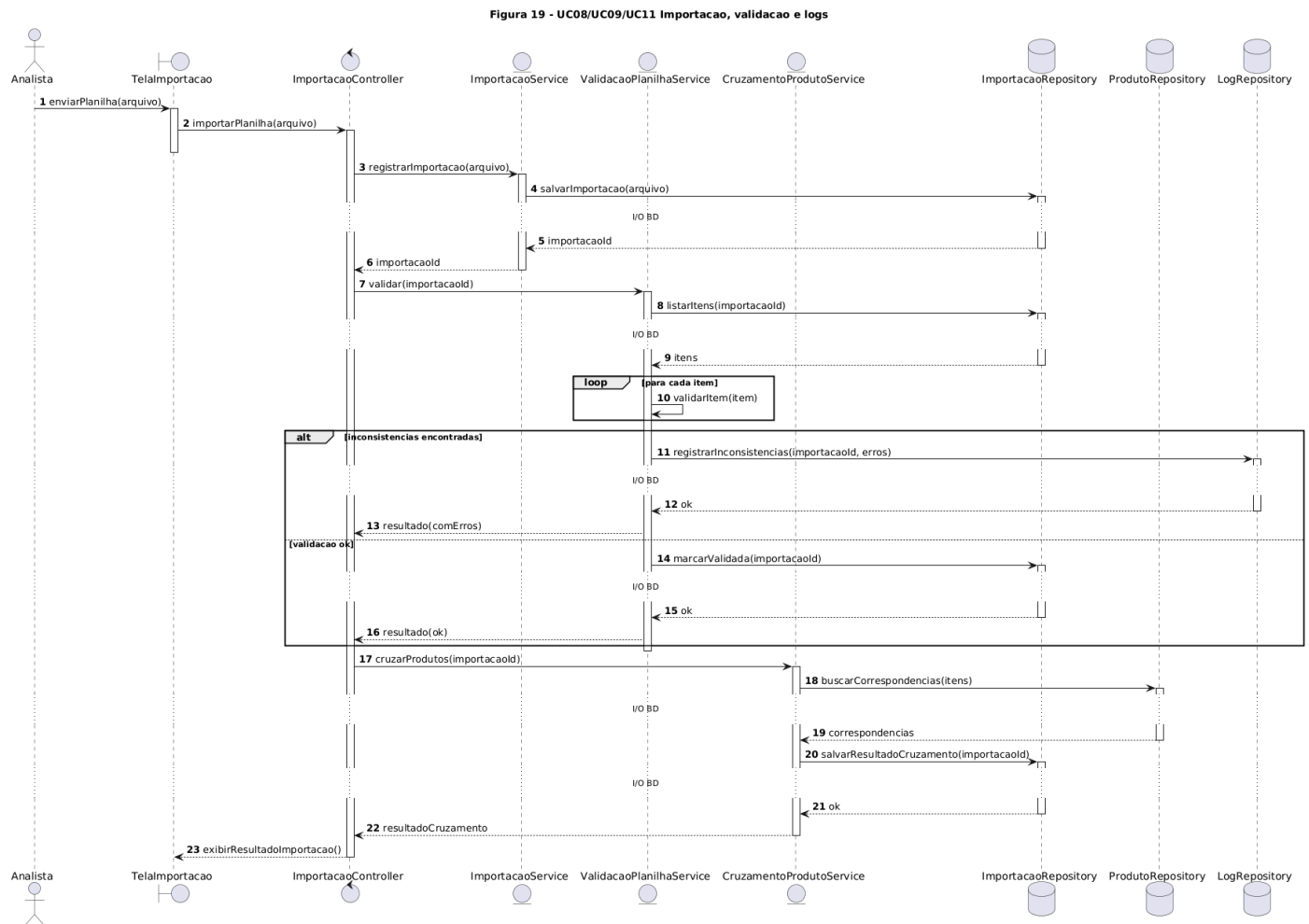
Figura 19. Diagrama de sequência de projeto – UC08/UC09/UC11
